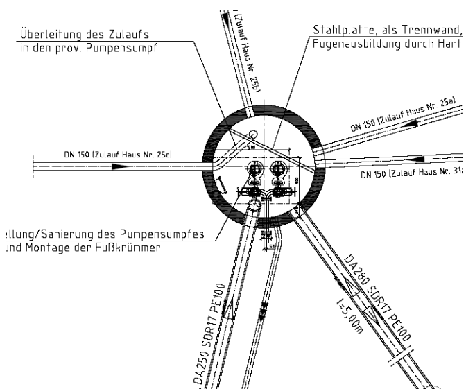
Pumpenaufstellung bei Umbau
